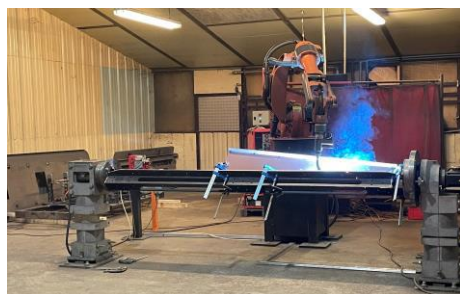
Robot de soudage KUKA Générateur Fronius TPS7000 1 vireur, capacité 2500 – 2 x 180°
